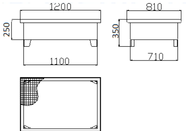
Ilustrační schéma – záchytná vana není vybavena roštem
